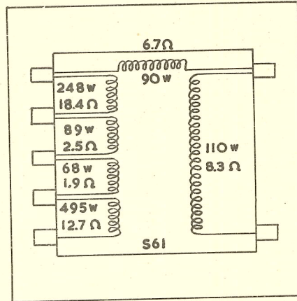
VOEDINGS TRAF0 GK 512 77
