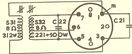
MFI SPOEL GK 56466
