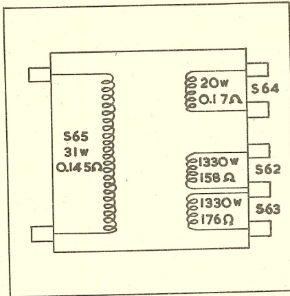
VOEDINGS TRAF0 GK 512 77
