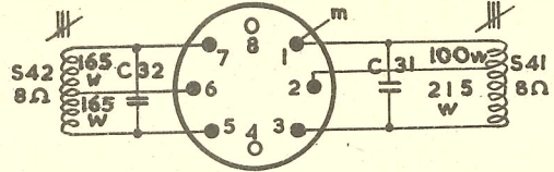
MFII SPOEL GK 56467
